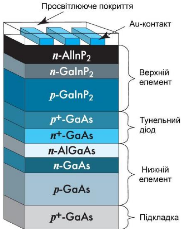
Рис.12. Каскадний елемент
