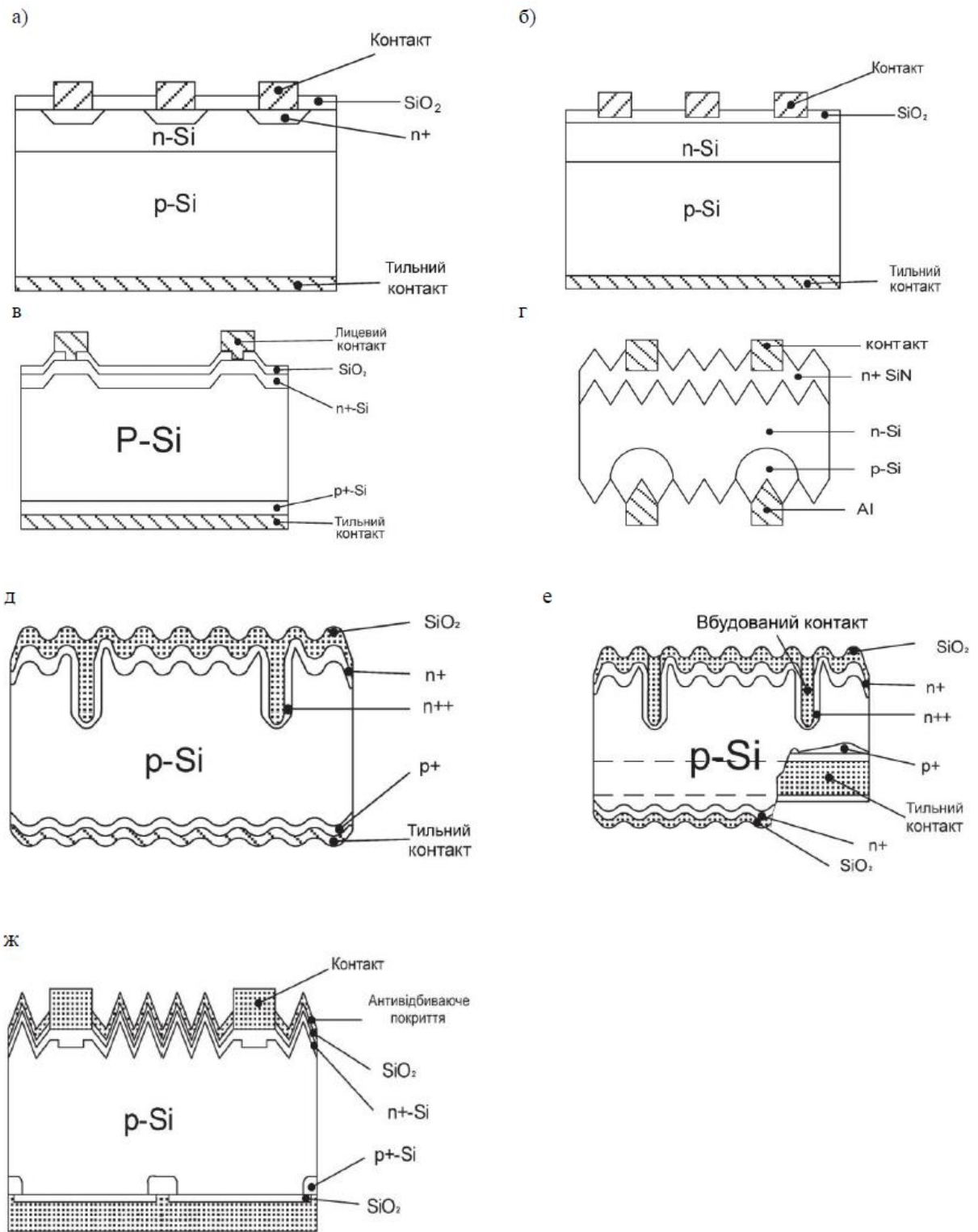
Рис. 6. Різні типи сонячних елементів на основі монокристалічного кремнію: а) простий р-п-перехід б) метал-ізолятор-п-р-структура (MINP) в) сонячний елемент із пасивуючим емітером (PESC) г) двошлицьовий сонячний елемент д) структура з однобічним вбудованим контактом (SSBS) е) структура із
