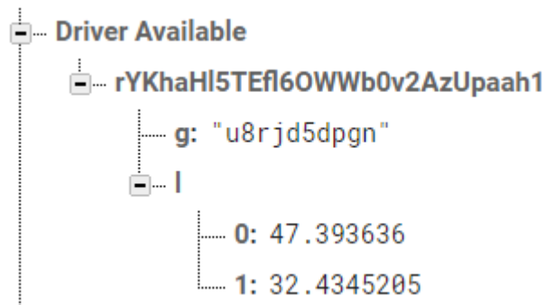
Рис. 2.7. Структура вузла «Driver Available»
