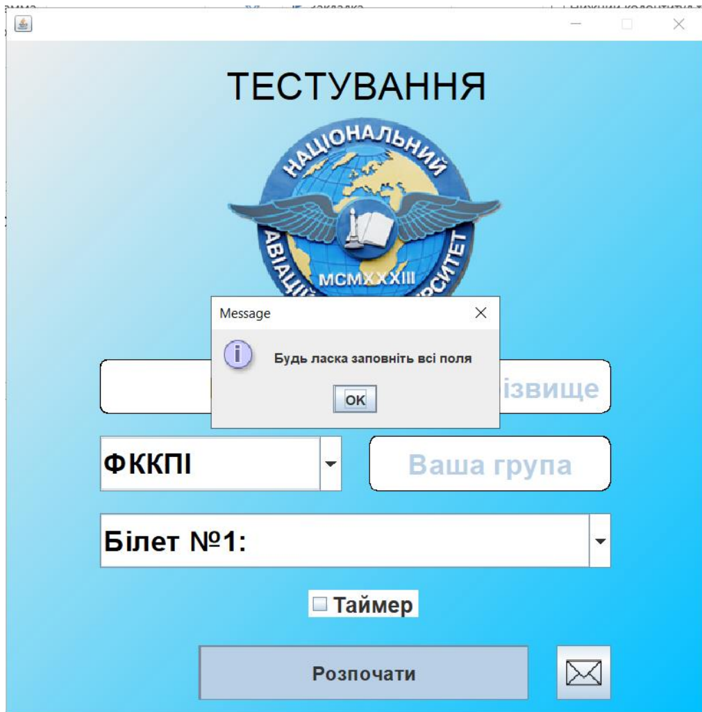
Рис. 3.6. Спливаюче повідомлення
