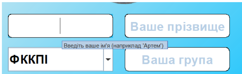
Рис. 3.7. Підказки
