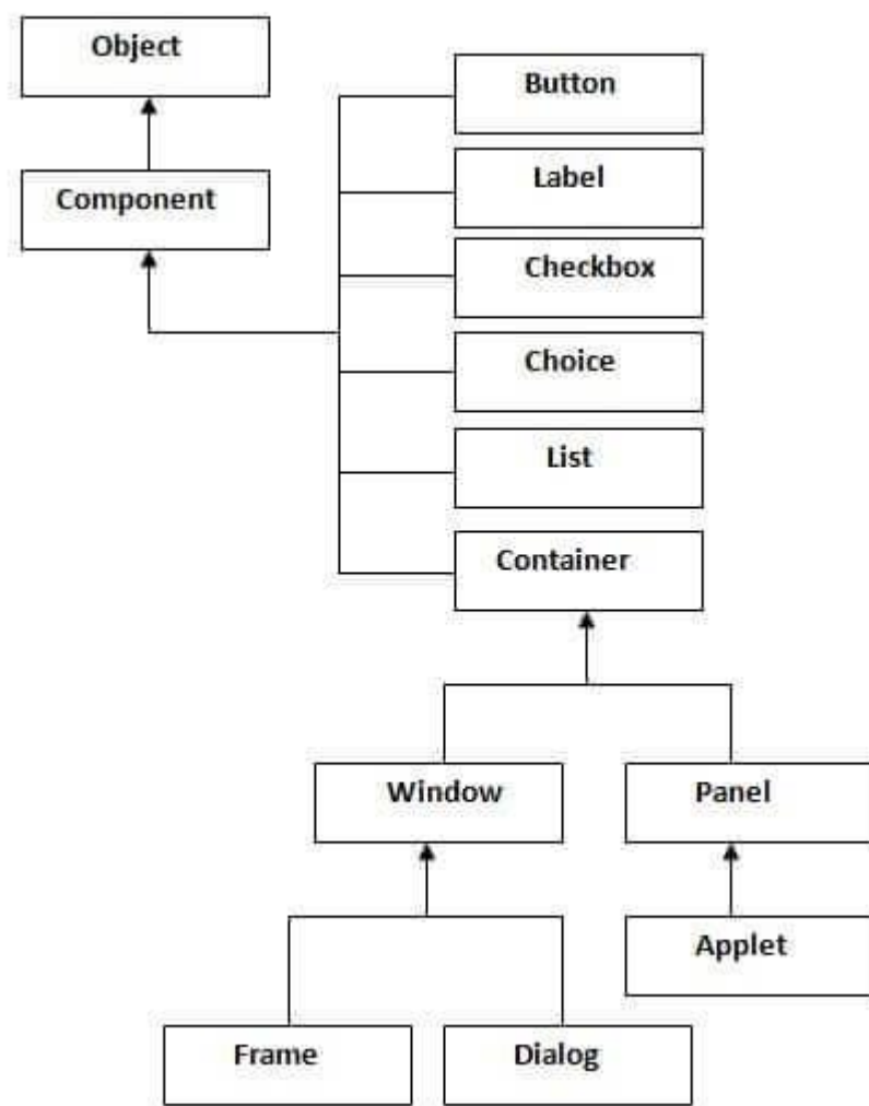
Рис. 2.3. Ієрархія класів Java AWT
