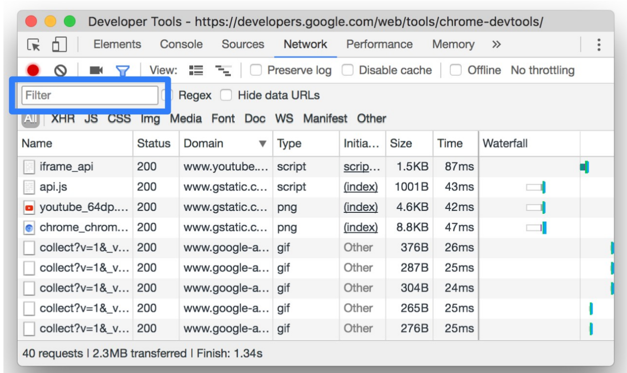
Рис 2.2 Фільтрування запитів
