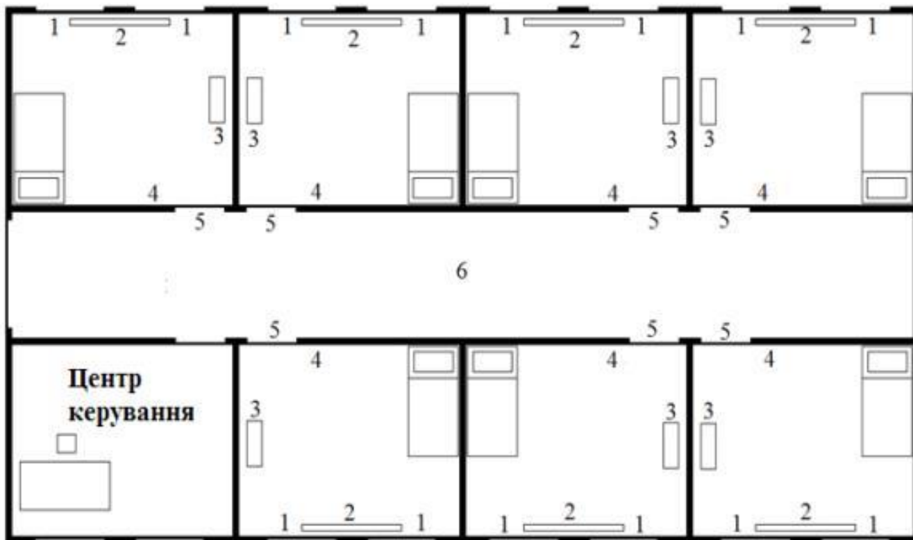
Рис. 5.3. Мережа з Wi-Fi маршрутизатором: 1 – сенсор контролю вікна; 2 – сенсор опалення; 3 – сенсор на кондиціонері; 4 – блок освітлення; 5 – точка доступу Bluetooth (шлюз); 6 – Wi-Fi роутер.
