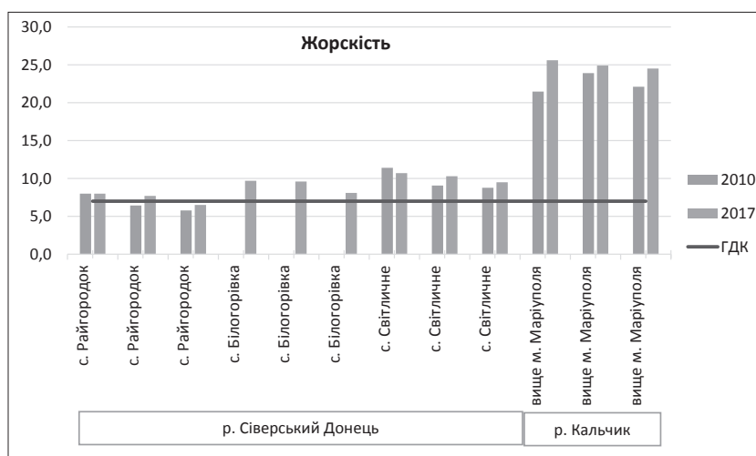
Рис. 7.13. Графічне подання даних моніторингу якості вод за показником жорсткість
