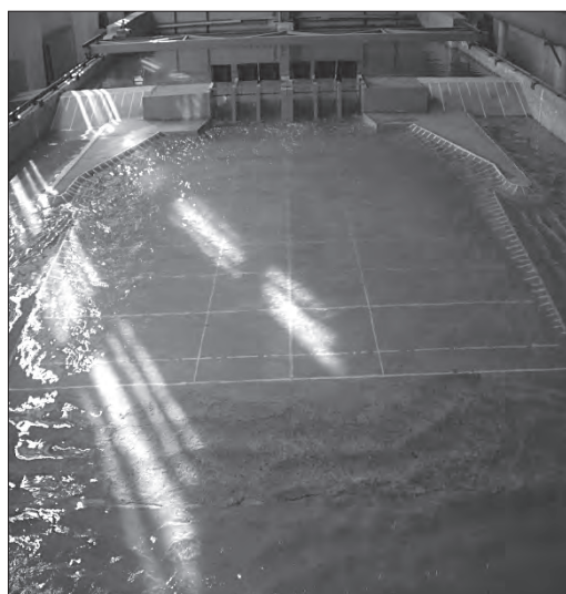
Фото 6.4. Лабораторні дослідження протипаводкової акумулюючої емкості на р. Тиса у Закарпатській області
