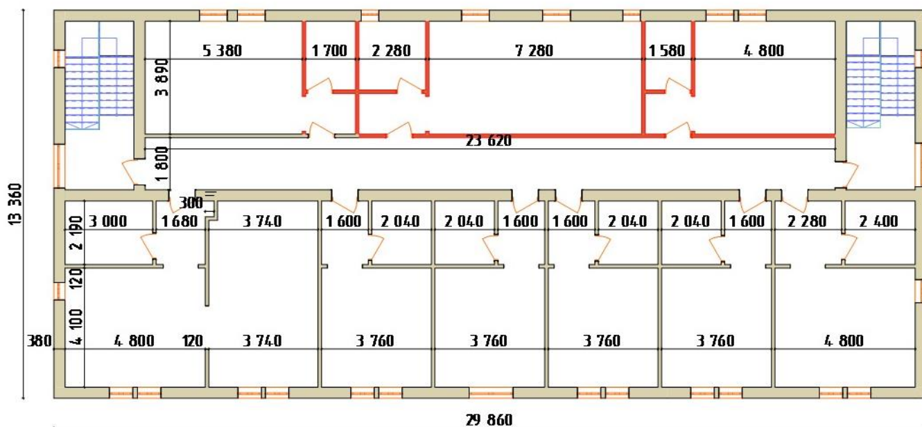
Рис. 3.3. План демонтажу типового поверху( 2-3 поверх) – червоним кольором позначені стіни які підлягають демонтажу.
