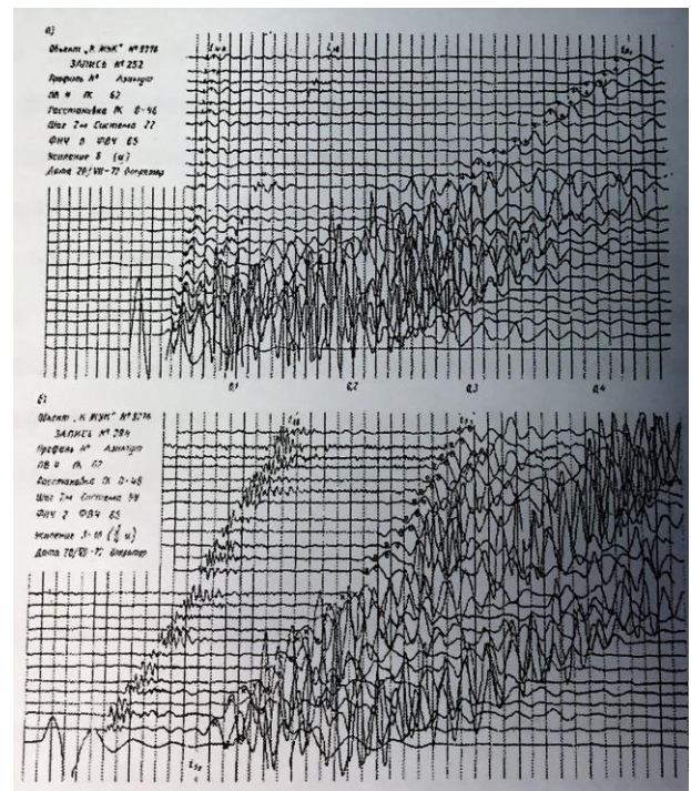
Приклад запису реальних поздовжніх (а) і поперечних (б) хвиль
