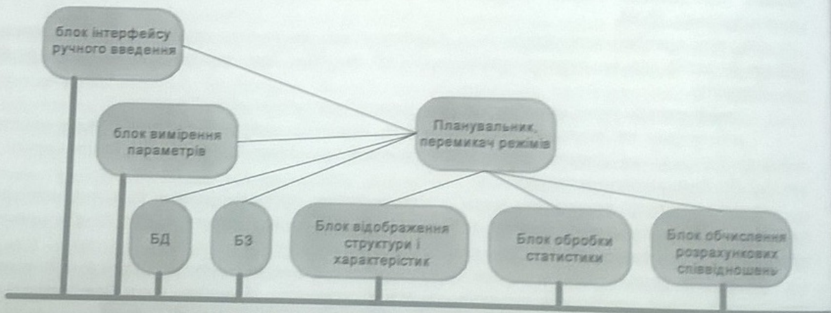
Мал. 2. Структура центрального блоку ПМА
