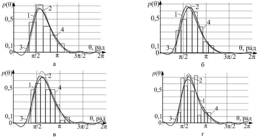
Рисунок 2 – Порівняння методу вибірових тригонометричних моментів та методу апроксимації емпіричних розподілів функціями Джонсона; обсяг вибірки: а – 30; б – 50; в – 70; г – 100
