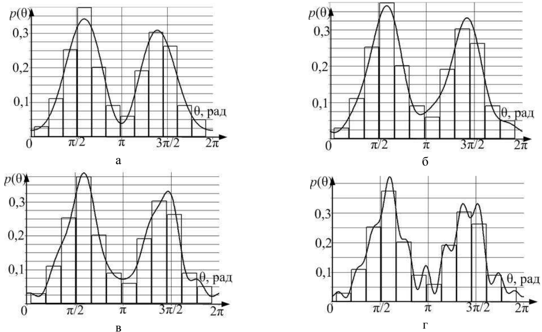
Рисунок 3 – Апроксимації двомодальної щільності ймовірності вибірки ВК; порядок найвищого використаного вибірового тригонометричного моменту: а – 3; б – 5; в – 9; г – 11
