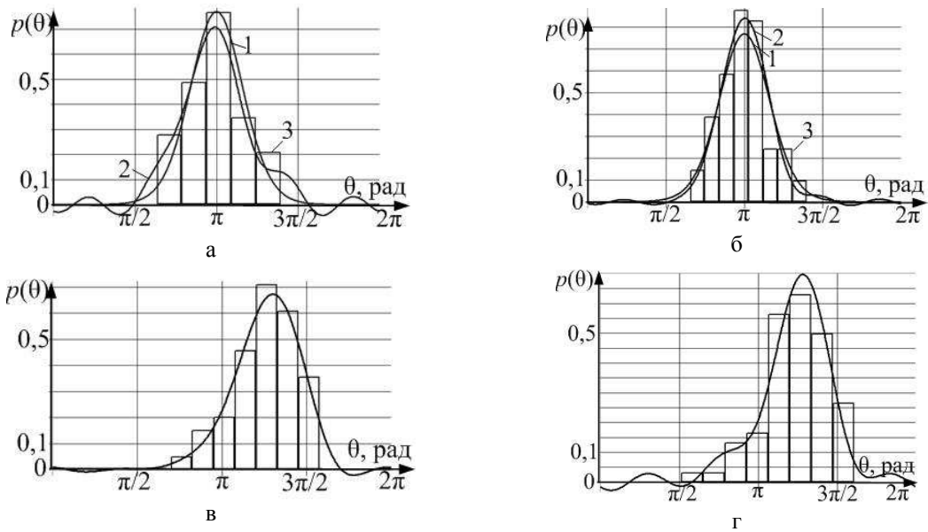
Рисунок 1 – Апроксимація вибірок ВК методом вибіркових тригонометричних моментів; обсяг вибірки: а – 30; б – 70; в – 50; г – 70
