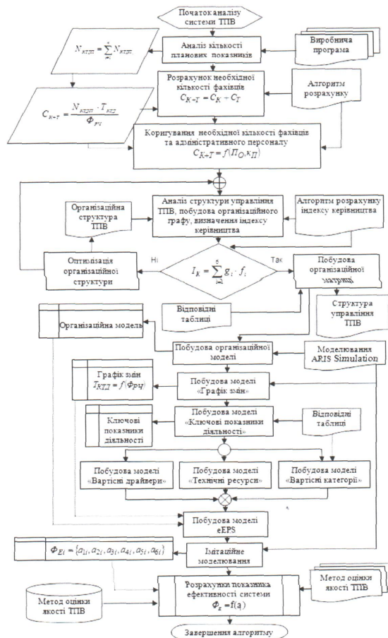
Рис. 3. Алгоритм методу аналізу та управління ефективністю ТПВ
