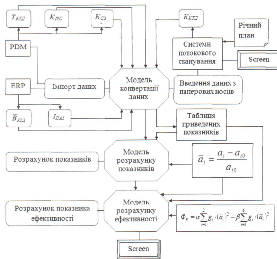
Рис. 4. Діаграма взаємодії програм розрахунку ефективності ТПВ
