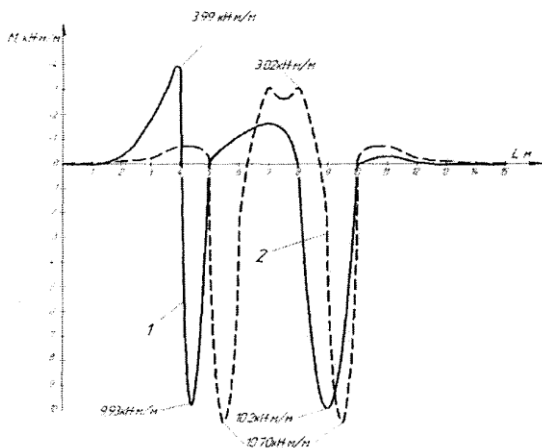
Рис. 7. Изгибающие моменты в покрытии от действия вертолета Ми-38 (монолитное покрытие): 1 – центральное нагружение; 2 – краевое нагружение
