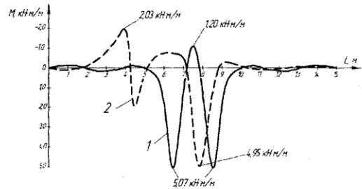
Рис. 4. Изгибающие моменты в покрытии от действия вертолета AW-139 (монолитное покрытие): 1 – центральное нагружение; 2 – краевое нагружение
