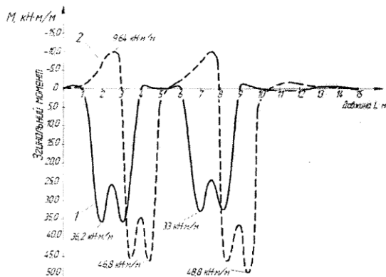
Рис. 6. Изгибающие моменты в покрытии от действия вертолета Ми-26 (монолитное покрытие): 1 – центральное нагружение; 2 – краевое нагружение
