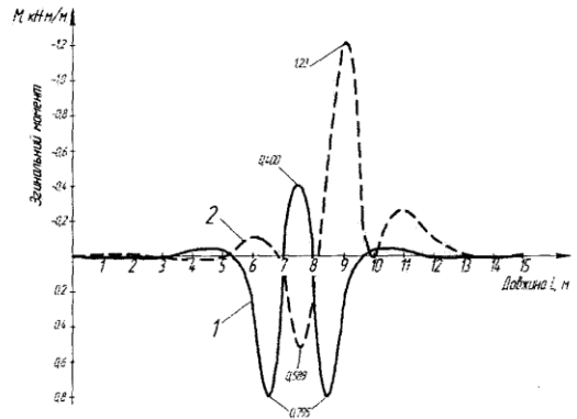
Рис. 5. Изгибающие моменты в покрытии от действия вертолета ЕС-155В1 (монолитное покрытие): 1 – центральное нагружение; 2 – краевое нагружение
