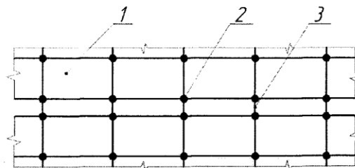
Рис. 1. Штыревые соединения между плитами покрытия в ПК ЛИРА: 1 – конечный элемент пластина; 2 – узел; 3 – конечный элемент № 55 (моделирует упругую связь между плитами покрытия)
