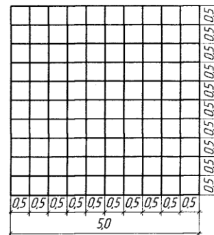
Рис. 2. Схема разбивки плиты покрытия на конечные элементы
