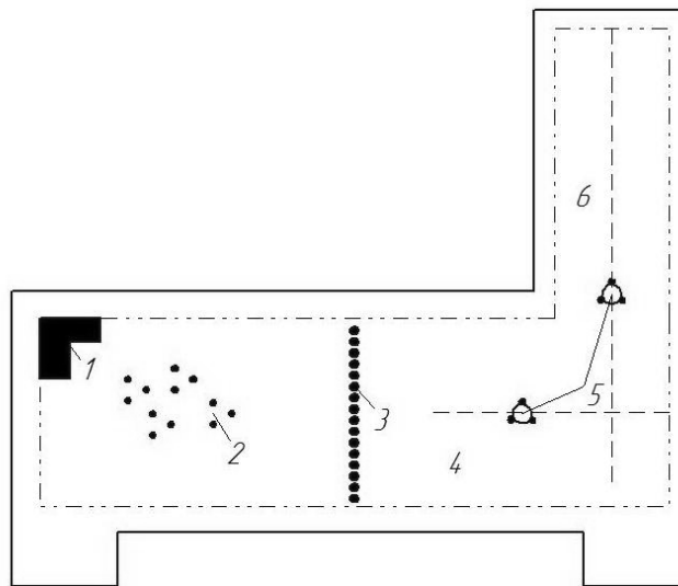
Рис. 1. – Схема планування вертодрому при Казанському вокзалі: 1 – службові приміщення; 2 – швартовочний майданчик; 3 – вогні, які позначають торець ЗПС; 4 – ЗПС1 розміром 60x25 м; 5 – зелений вогонь (центр ЗПС); 6 – ЗПС2 розміром 60x17м
