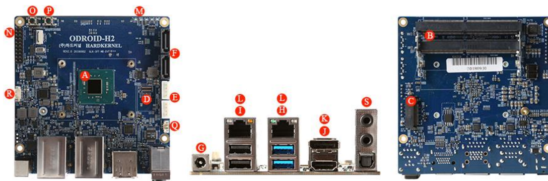
Рисунок 2.8 – Мікрокомп’ютер Odroid H2
