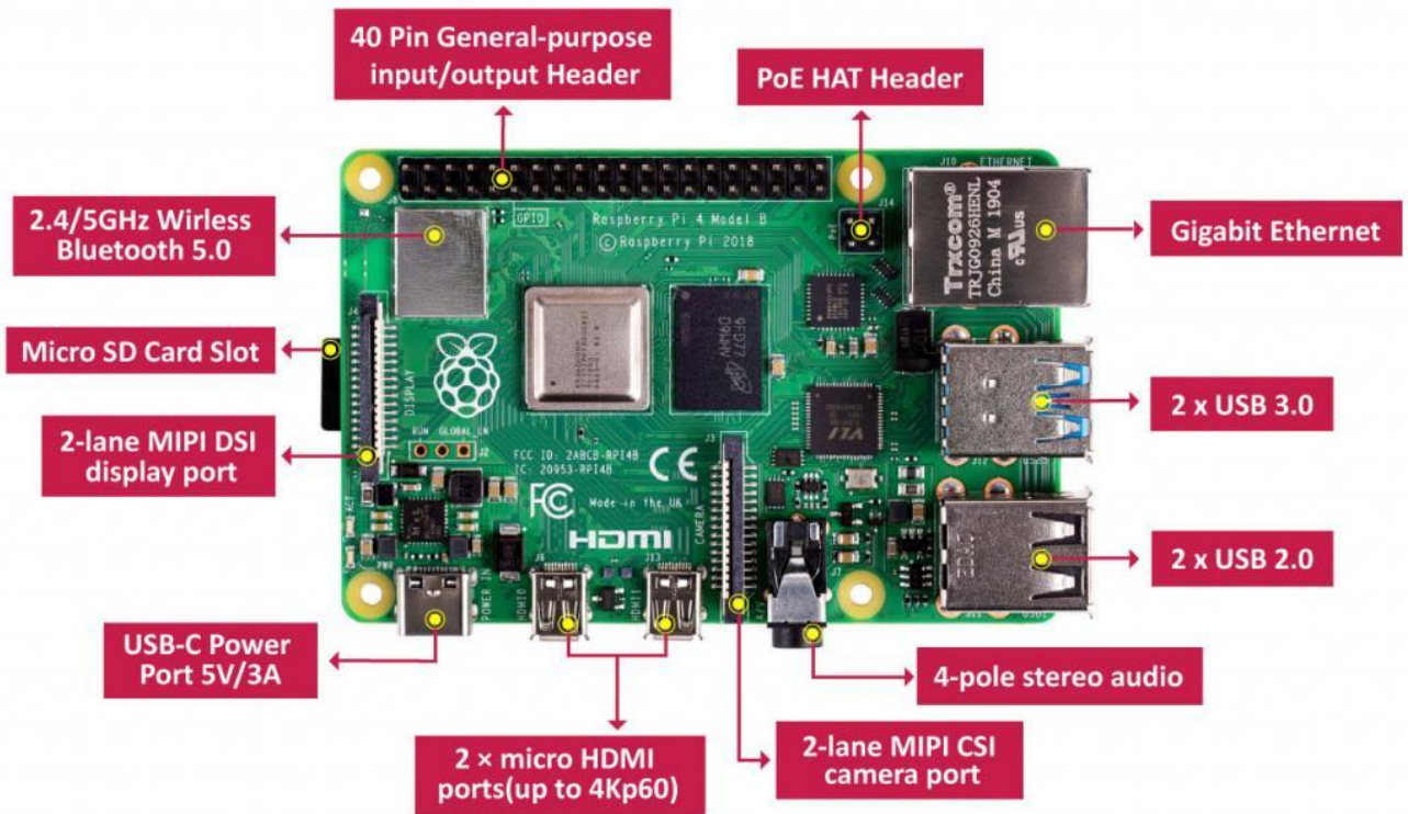
Рисунок 2.1 – Мікрокомп'ютер Raspberry Pi 4 Model B
