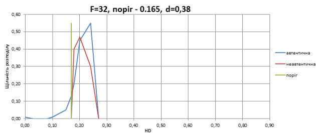
Рис. 4.2. Полігони частот відстаней Хеммінга для різних фільтрів
