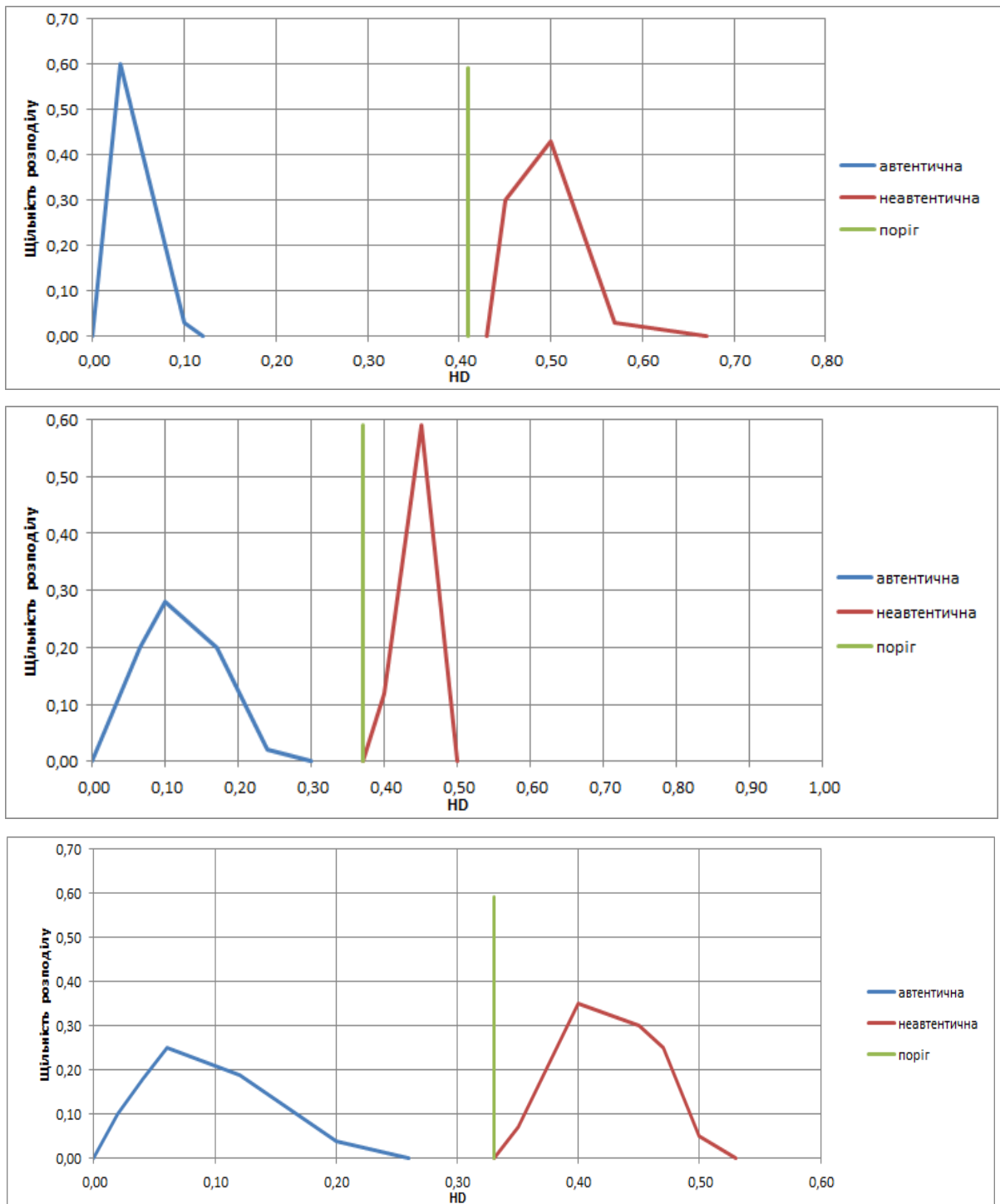
Рис. 3.7 Полігони частот для райджок, що належать різним людям. Значення порогів, визначені за критерієм Неймана-Пірсона показані чорної суцільною лінією
