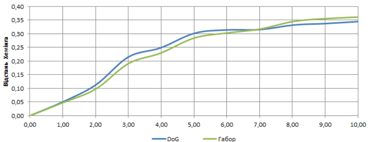
Рис. 3.5 Чутливість відстані Хеммінга до нахилу голови для фільтрів Габора ( \omega_0 = \pi/8, \theta = 0 ), і DoG-фільтра ( \sigma = 0,1 ). Кут (Angle) показаний в градусах
