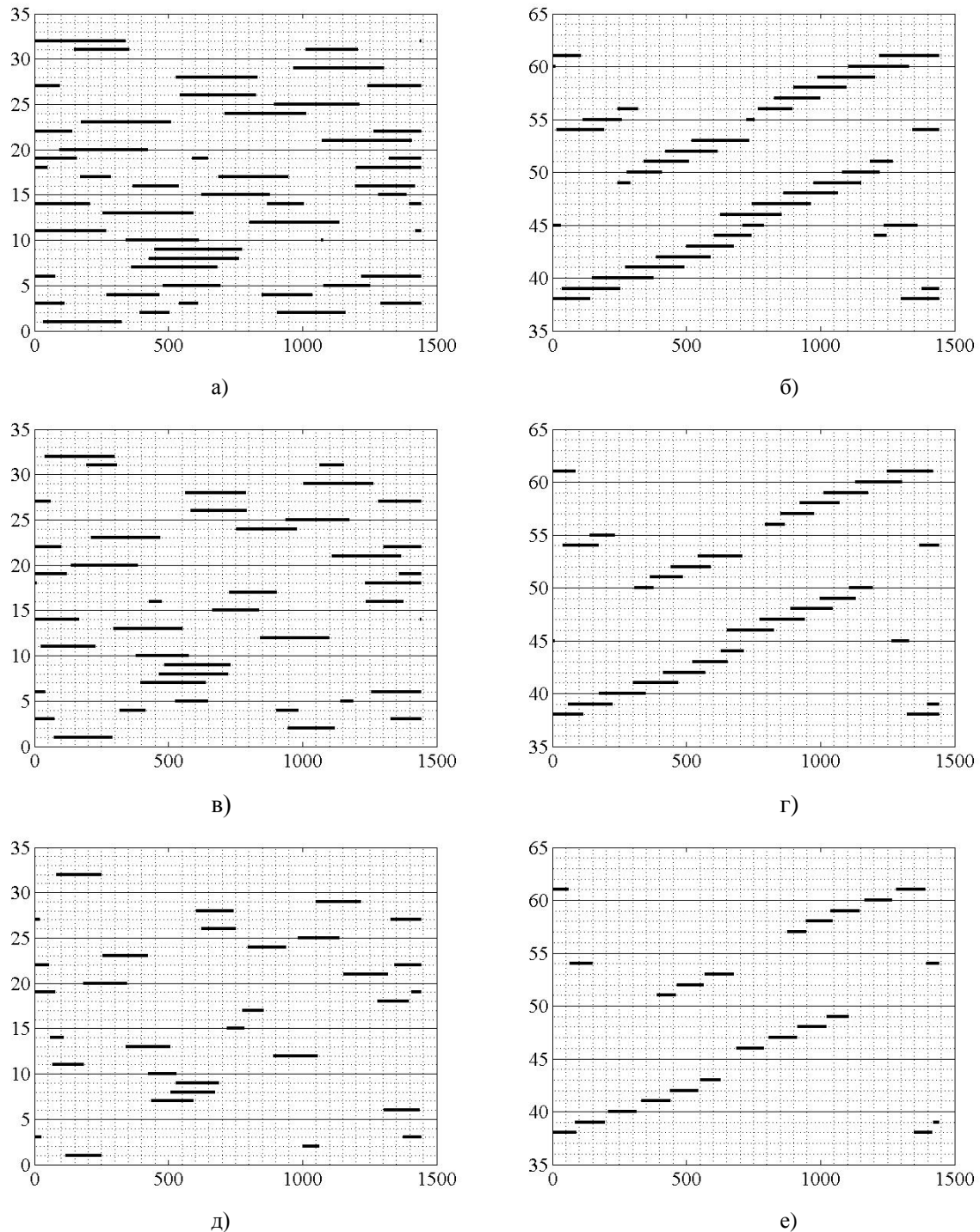
Рис. 4. Диаграммы доступности спутников: а) – GPS (высота 3000 км, угол видимости 10^\circ ), б) – ГЛОНАСС (высота 3000 км, угол видимости 27^\circ ), в) – GPS (высота 4000 км, угол видимости 24^\circ ), г) – ГЛОНАСС (высота 4000 км, угол видимости 37^\circ ), д) – GPS (высота 6000 км, угол видимости 40^\circ ), е) – ГЛОНАСС (высота 6000 км, угол видимости 48^\circ )
