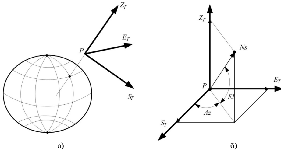
Рис. 1. Топоцентрическая система координат: а) – расположение осей относительно Земли б) – положение спутника N_s относительно осей
