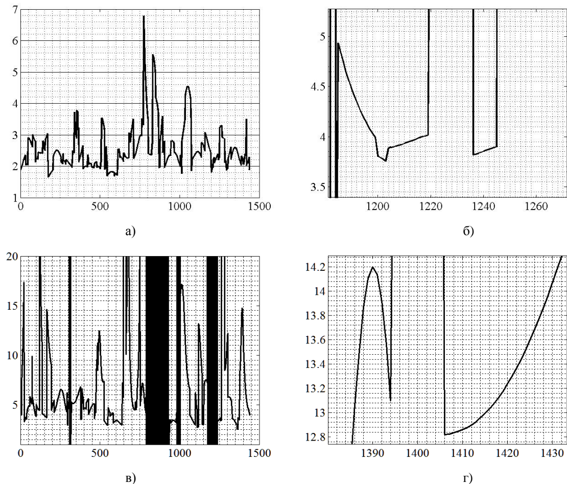
Рис. 5. Пространственно-временной геометрический фактор ( GDOP ): а) – GPS (высота 3000 км, угол видимости 10^\circ ), б) – ГЛОНАСС (высота 3000 км, угол видимости 27^\circ ), в) – GPS (высота 4000 км, угол видимости 24^\circ ), г) – GPS (высота 6000 км, угол видимости 40^\circ )
