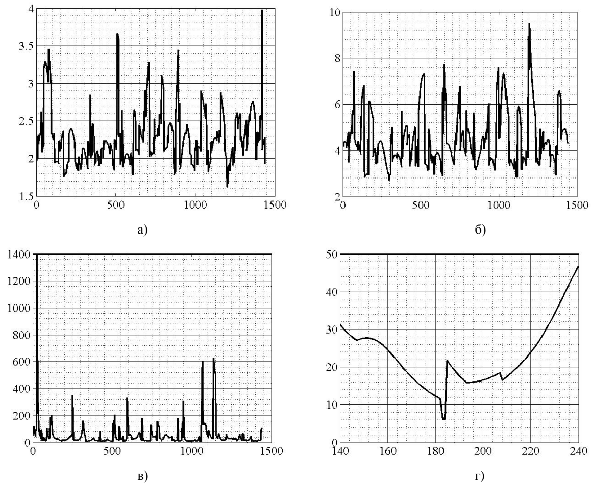
Рис. 6. Пространственно-временной геометрический фактор (GDOP) при объединенных GPS и ГЛОНАСС: а) – высота 3000 км, угол видимости 10^\circ , б) – высота 4000 км, угол видимости 24^\circ для GPS и 37^\circ для ГЛОНАСС, в) – высота 6000 км, угол видимости 40^\circ для GPS и 48^\circ для ГЛОНАСС, г) – высота 6000 км, угол видимости 40^\circ для GPS и 48^\circ для ГЛОНАСС, диапазон временных отсчетов 140-240 минут
