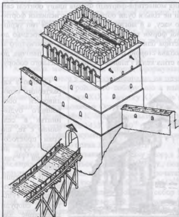
Рис. 1. Надбрамна башта Дерманського монастиря. Аксонометрія. Вигляд із північного сходу. Реконструкція станом на XV ст.
